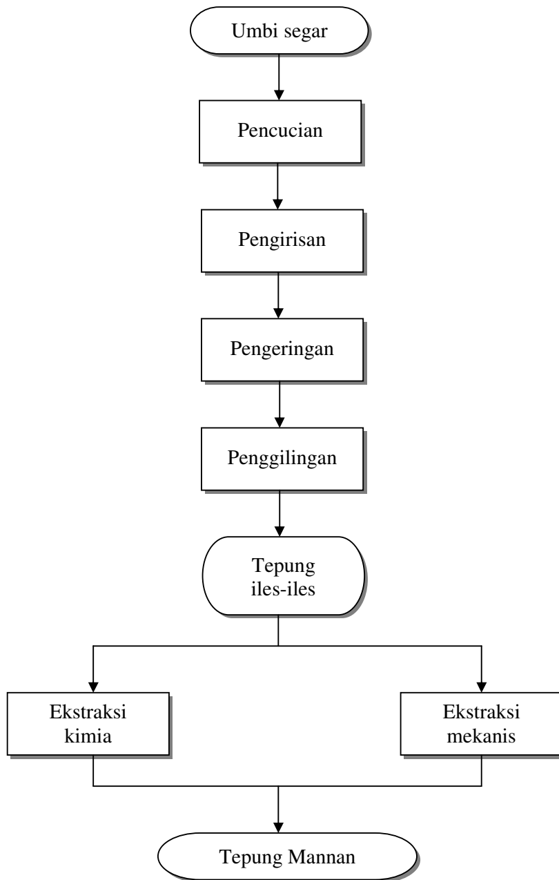
Gambar 1. Diagram alir proses pembuatan tepung mannan (BPK, 1977)
